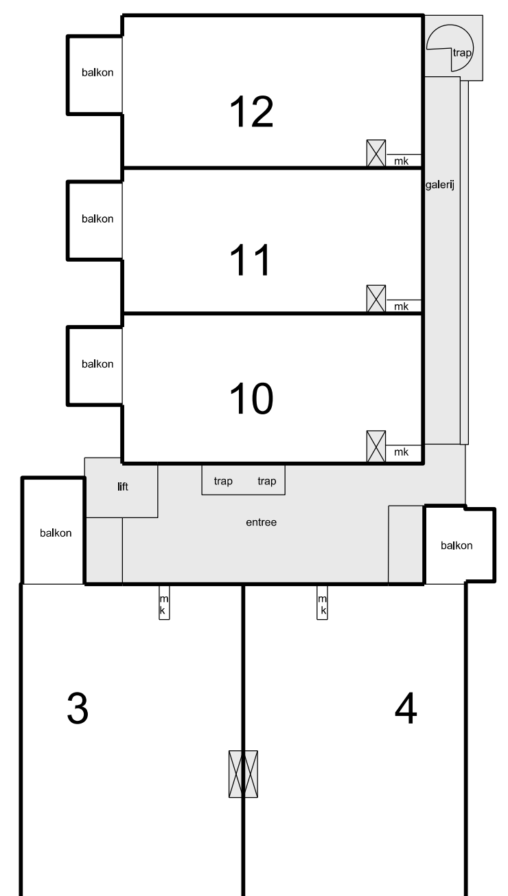
1 e verdieping 1 : 200
