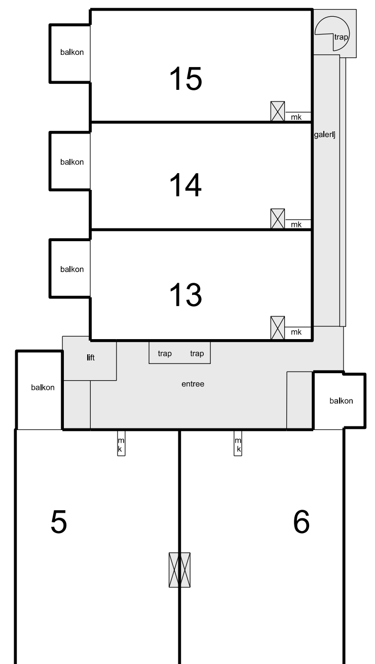
2 e verdieping 1 : 200
